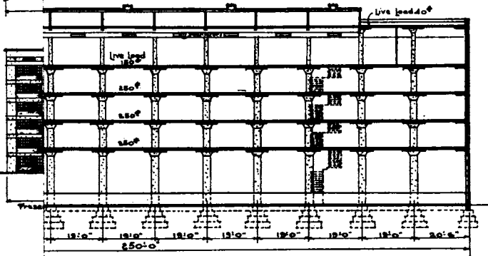
Longitudinal Section —
